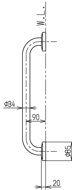
取付座詳細(1:2)
